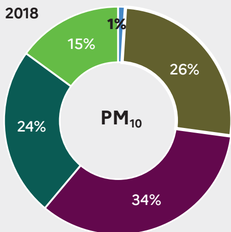
Répartition des émissions en particules fines (PM10 et PM2,5) en France (Métropole)
